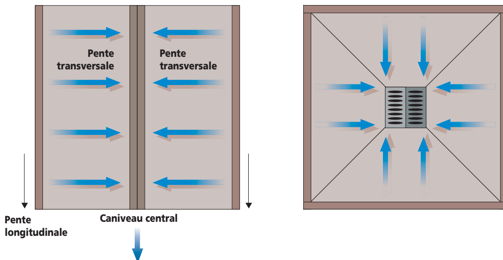
Figure 12: exemples de systèmes de collecte des eaux superficielles.
