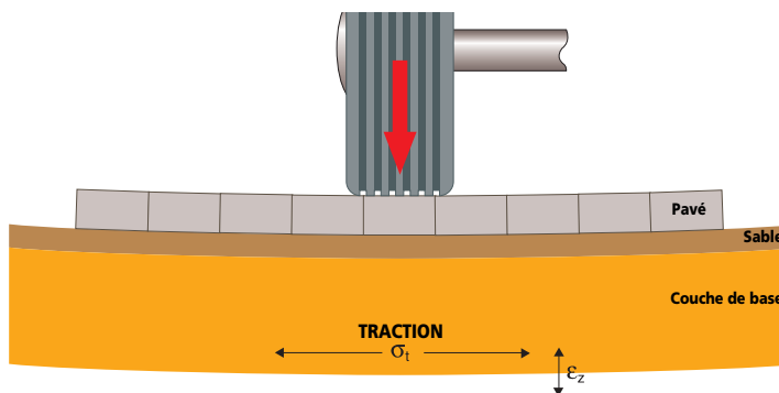
Figure 14 : principe de dimensionnement dans le cas d'assise rigide.
