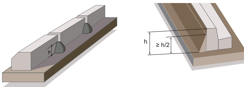
Figure 21 : calage d'une bordure par épaulement et par solin continu.
