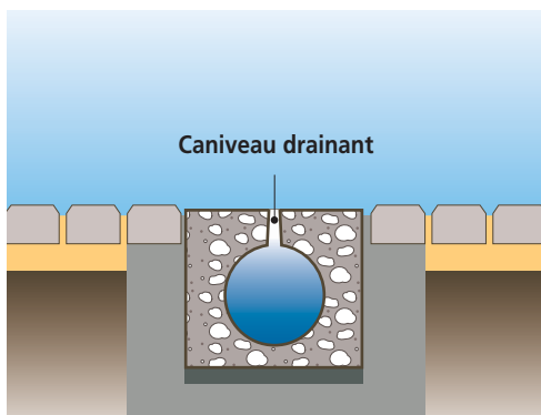
Figure 27 : caniveau drainant à fente.
