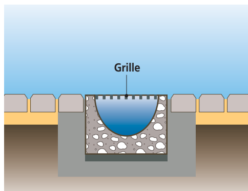
Figure 28 : caniveau drainant à grille.
