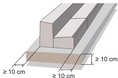
Figure 20: caractéristiques minimales du massif de fondation.
