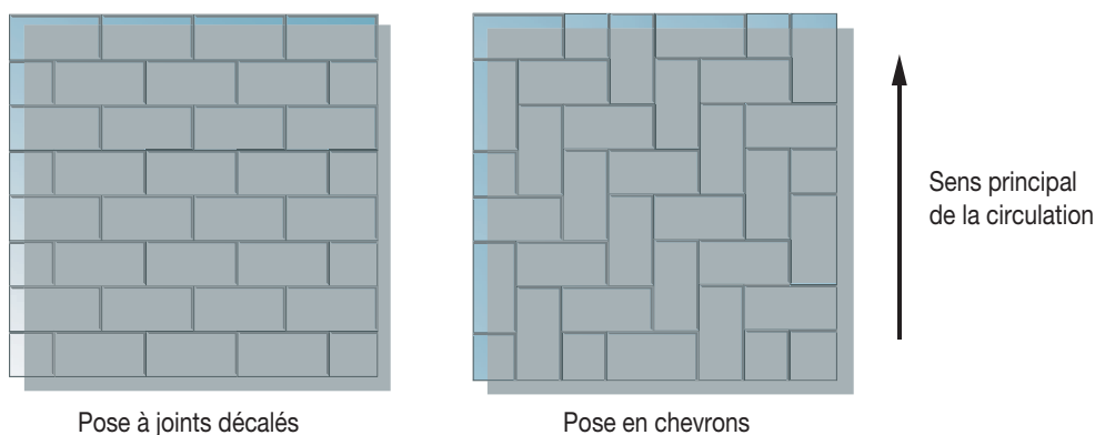
Figure 15: exemple d'appareillage pavés
