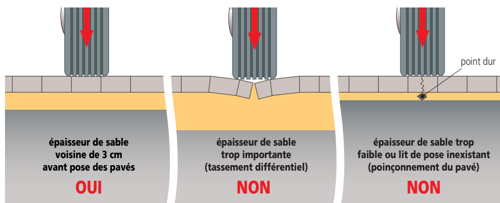
Figure 24 : dispositions constructives pour lit de pose.
