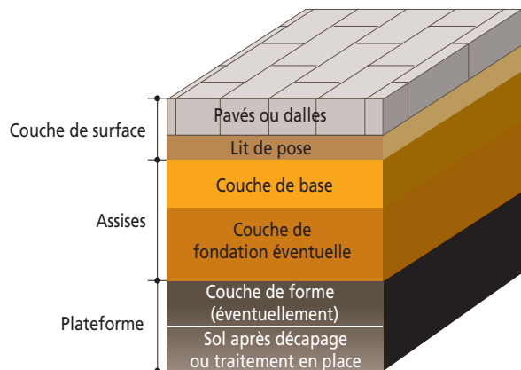
Figure 11 : exemple de structure de chaussée.
