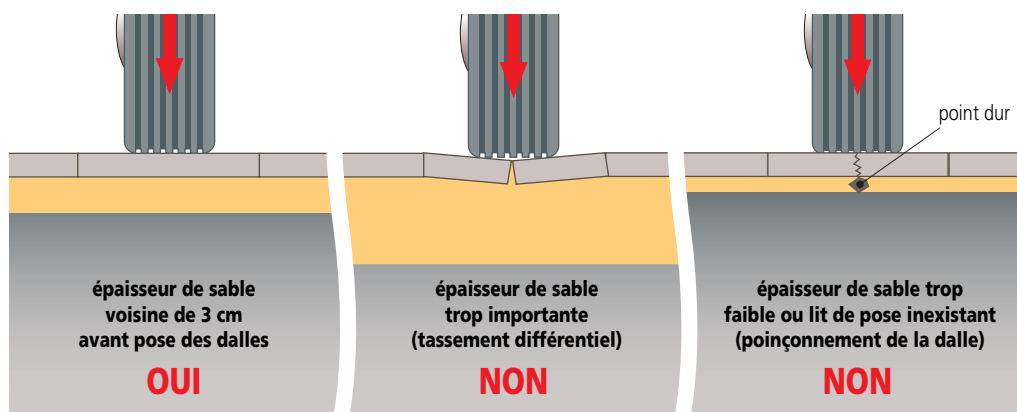
Figure 29: dispositions constructives pour lit de pose.
