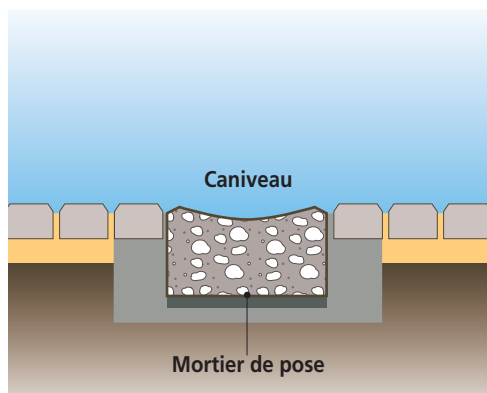
Figure 26: caniveau préfabriqué
