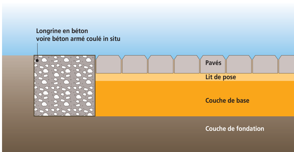
Figures 22 et 23 : exemples de blocage de rives.
