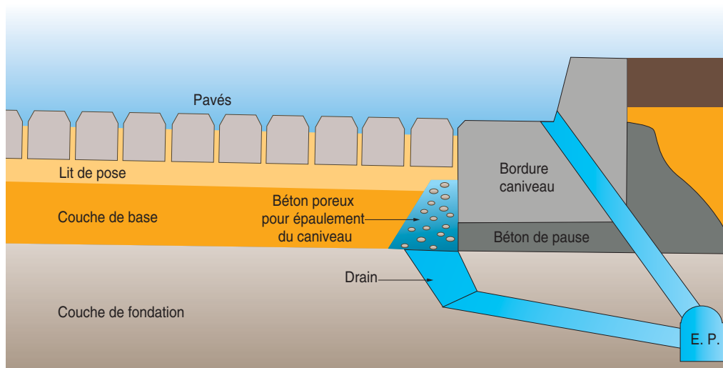
Figure 30: exemple de dispositif de drainage.
